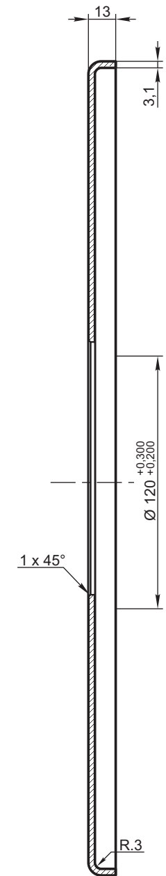
CORTE A-A
