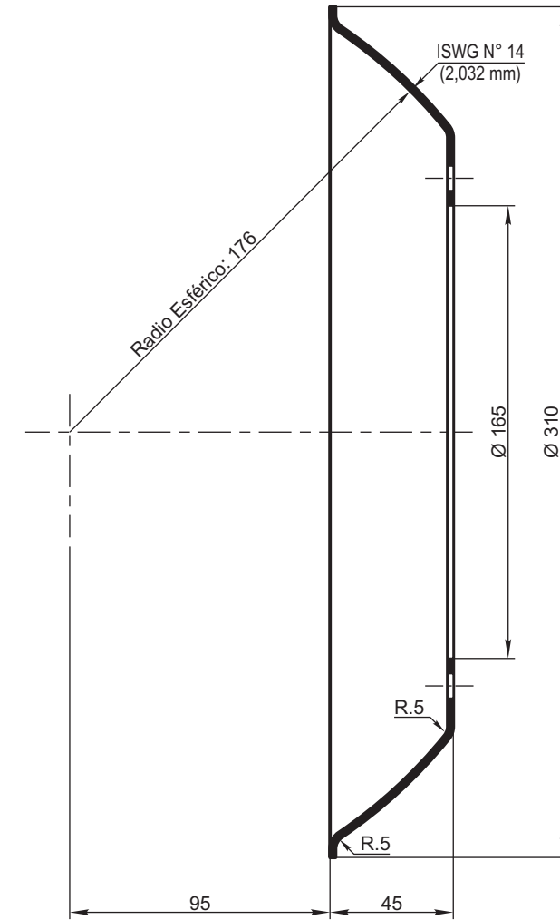
CORTE A-A
