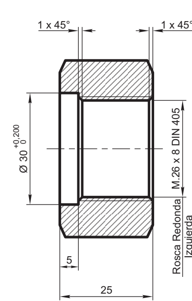
CORTE A-A
