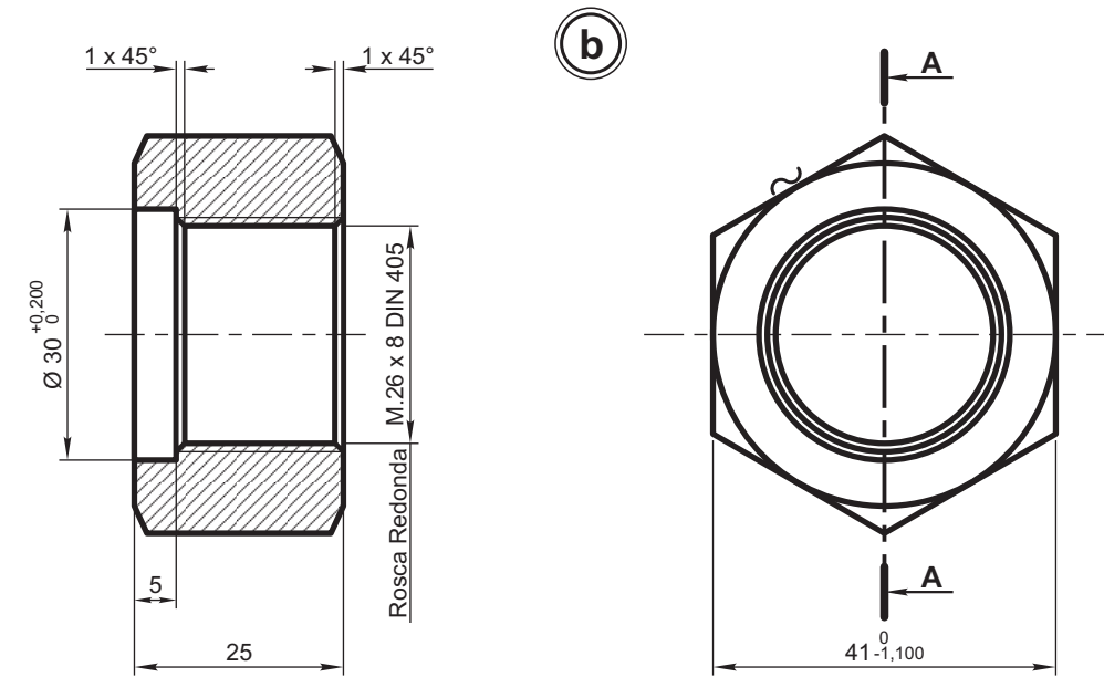
CORTE A-A
