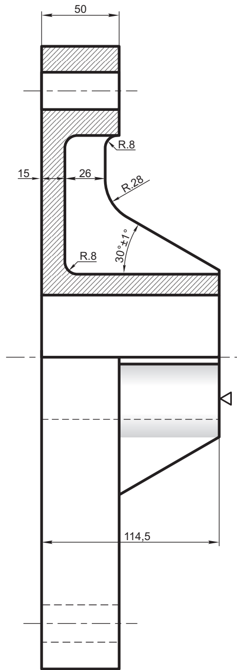
CORTE A-A
