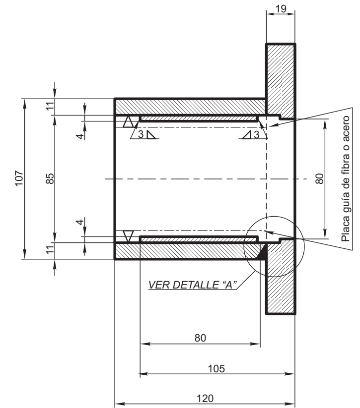
CORTE B-B
