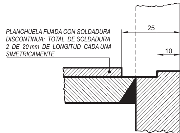
Detalle A Esc. 1:1
