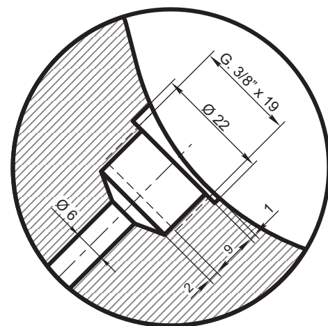
DETALLE B
