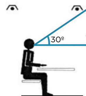
Situación de las luminarias en función del ángulo de visión.
