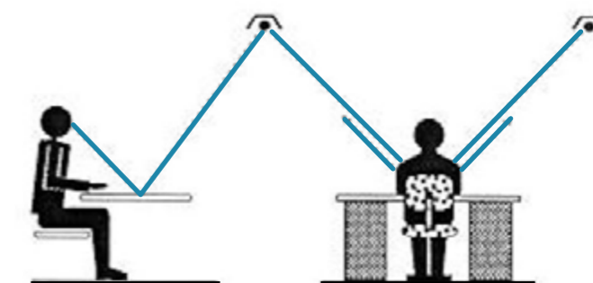
Situación de las luminarias en relación con el ángulo de reflexión de la superficie de trabajo Izq.: Disposición deficiente de luminarias: la luz reflejada coincide con la línea de visión. Der.: Disposición correcta de luminarias: la luz reflejada no coincide con la línea de visión.
