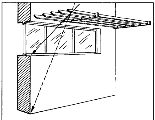
Figura 83.e Un toldo hecho de hileras de tablillas ofrece una protección buena contra la penetración del calor y mejores condiciones de iluminación que un toldo continuo, sin rendijas
