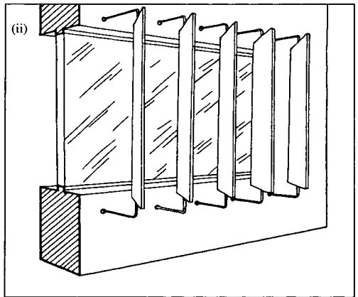
Figura 83d. Pantallas verticales exteriores contra la radiación solar. (i) Fijas. (ii) Regulares
