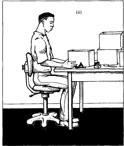
Figura 15a. (i) y (ii) Reduzca la distancia entre el trabajador y el objeto de trabajo
