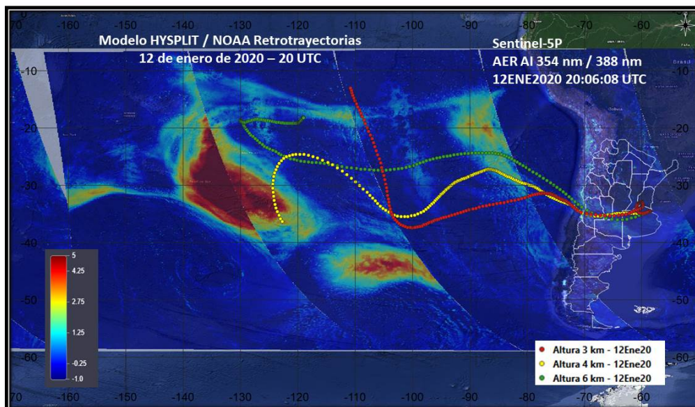
Figura 3. Medición del Índice de Aerosol (AI) y retrotrayectorias HYSPLIT/NOAA para el 12 de enero de 2020.
