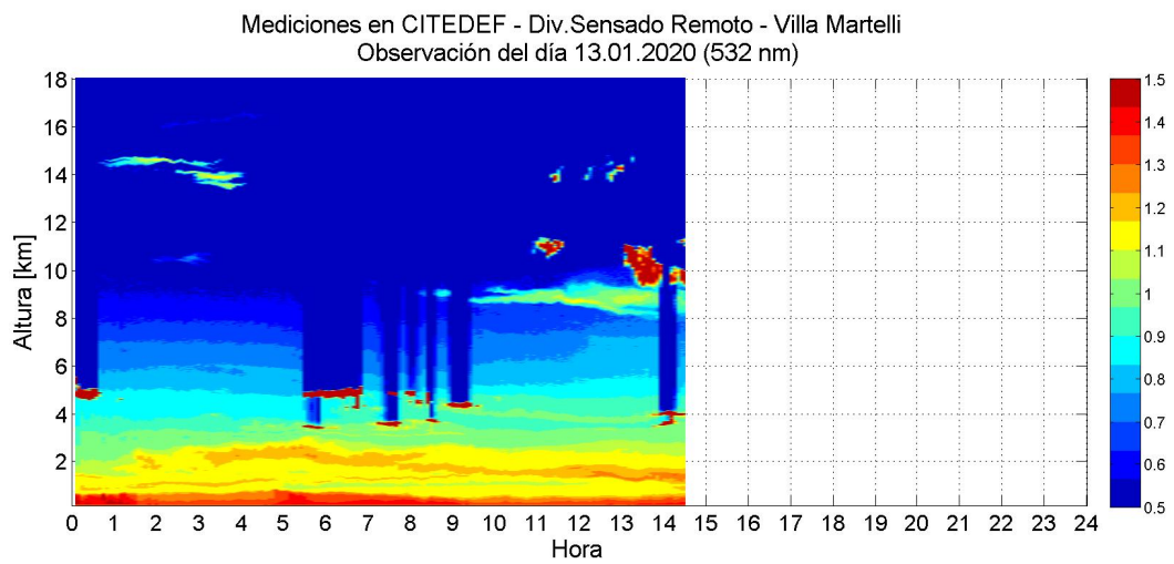
Figura 2. Medición LIDAR en 532 nm para el 13 de enero de 2020.
