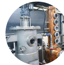
Planta piloto compacta para la generación de bioetanol
