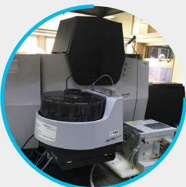
Espectrofotometro de absorción atómica para determinación de metales en alimentos, efluentes, fertilizantes y minerales
