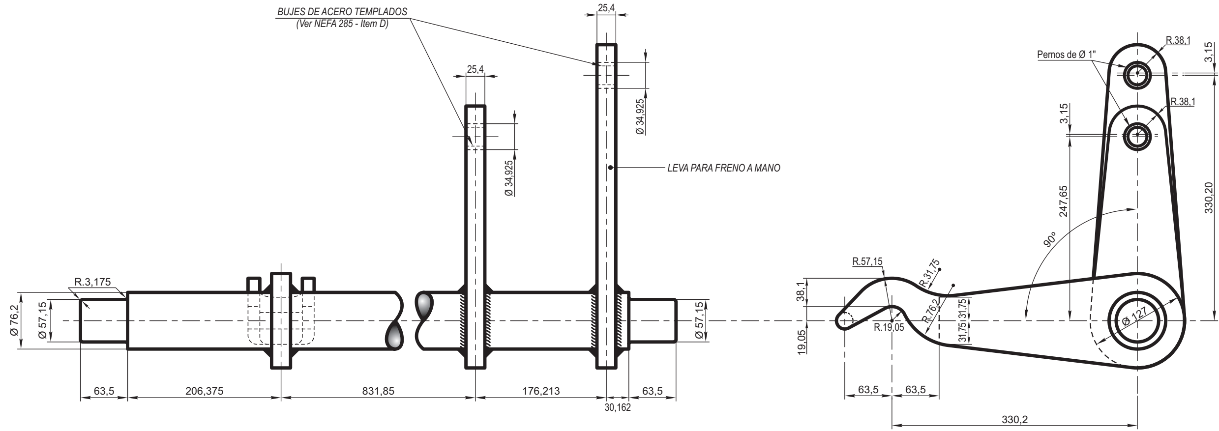
PIEZA N° 826/A y PIEZA N° 826/B
