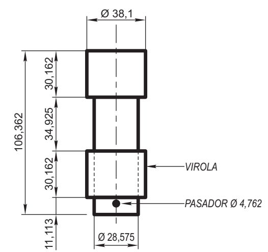
PERNO CEMENTADO Y TEMPLADO PIEZA N° 826/C*
