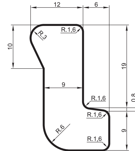
ARO "GIBSON" TIPO STANDARD Esc. 2:1
