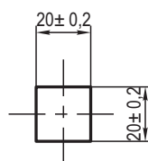
CORTE A-B
