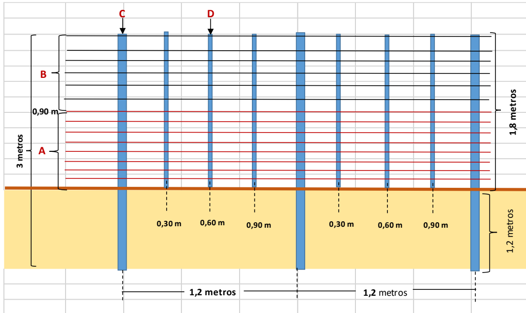
Figura 1: Esquema del alambrado
