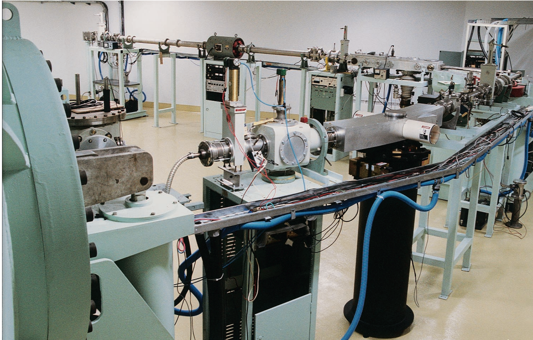
| Línea de alta energía del acelerador (diciembre 2000)
