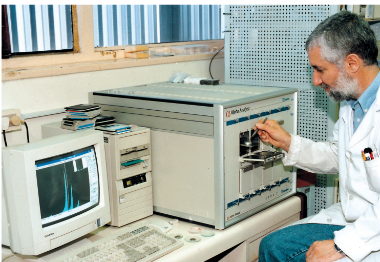
Sistema de medición de muestras ambientales por espectrometría alfa
