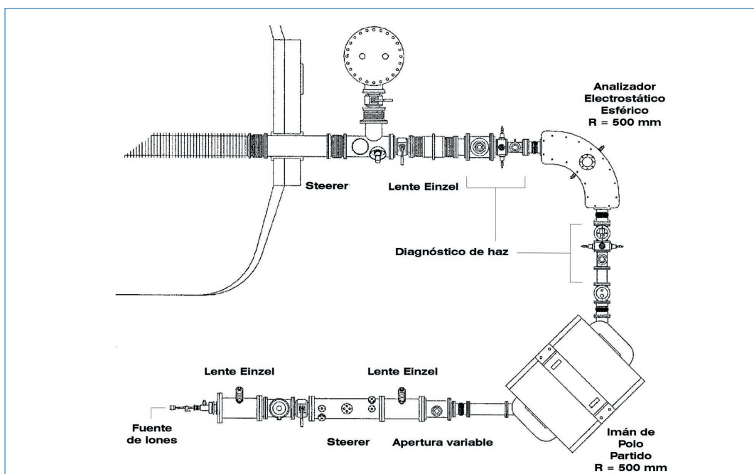
Figura 23. Esquema de la línea de inyección del acelerador
