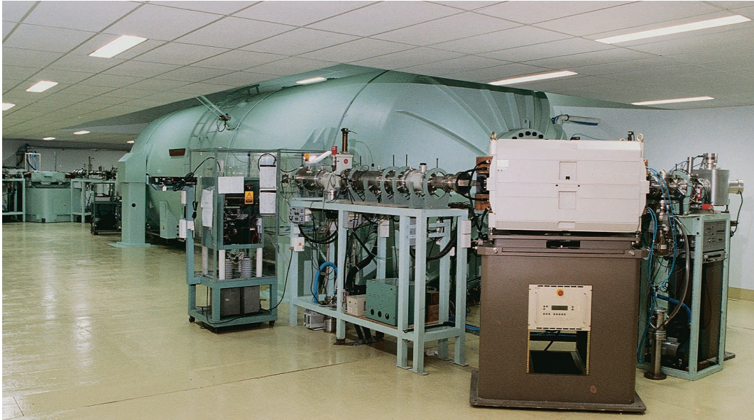
Espectrómetro de masas con acelerador (diciembre de 2000)
