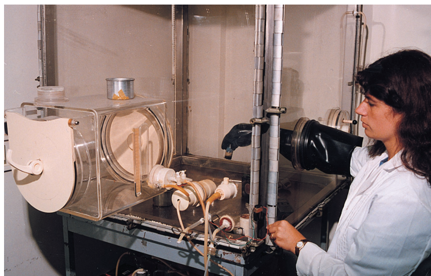
Cámara de referencia para la calibración de detectores de radón en el aire
