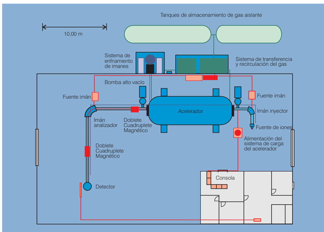
Figura 22. Esquema del Centro de Espectrometría de Masas con Acelerador
