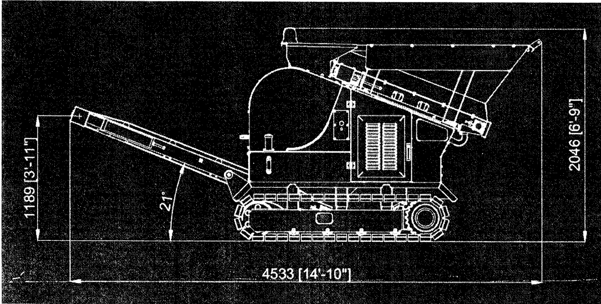
a) Medidas de la Trituradora Largo
