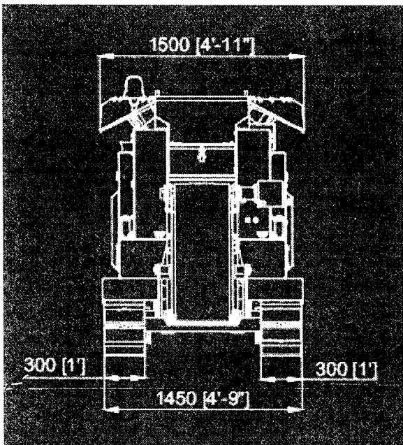
a) Medidas de la Trituradora en Ancho
