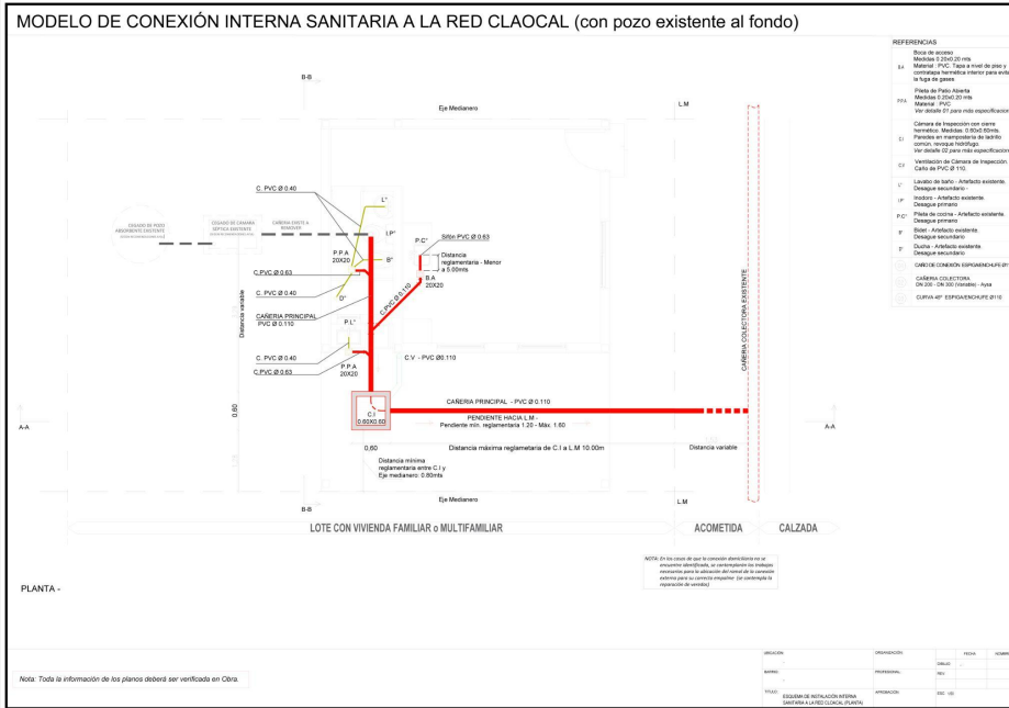
ESQUEMA DE CONEXIÓN INTERNA SANITARIA A LA RED CLOACAL (con pozo existente al fondo)
