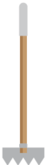
MCLEOD O RASTRILLÓN Largo 125 cm Peso 2.3 Kg.
