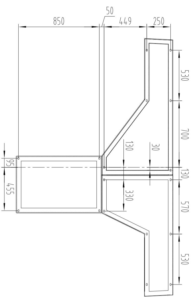
Diagrama esquemático de la posición de agujeros de montaje de pernos de la parte interior del panel de control
