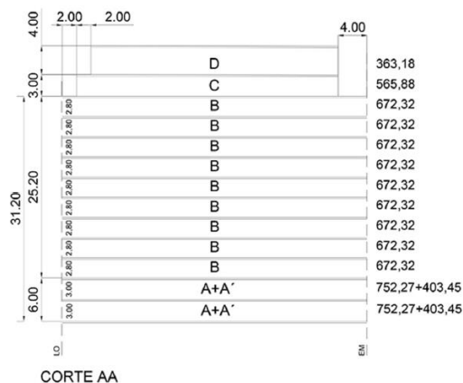
CORTE AA
